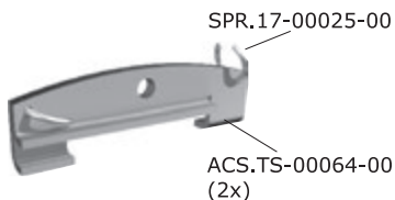
Sicherungsbügel für Zargenhaken securing element for hooks, 120g
