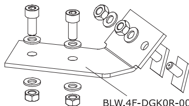
Konsole rechts bracket right
