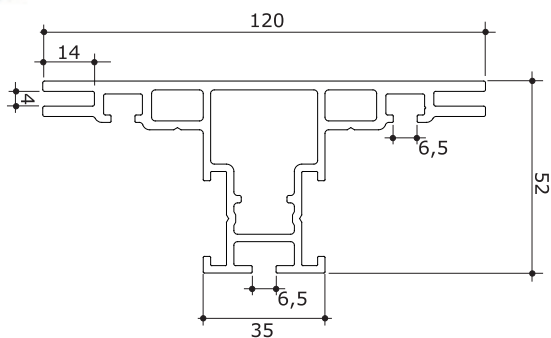
Rahmenprofil für 3mm Flach-Keder profile for frames and 3mm flat keder 1000mm - 2460g, Herstellungslänge 6100mm production length is 6100mm
