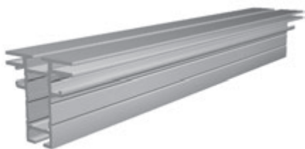
Rahmenprofil für 3mm Flach-Keder profile for frames and 3mm flat keder, 1000mm - 1367g, Herstellungslänge 6100mm production length is 6100mm
