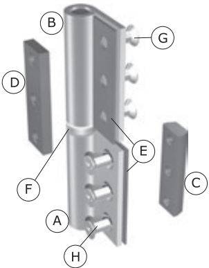
Scharnier für Anschlagtür DIN links hinge for door DIN left
