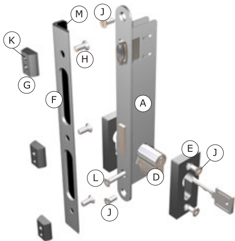
Schloss komplett für Universaltür, 3 Schlüssel complete lock for universal door, 3 keys
