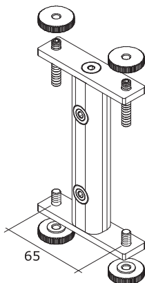
Abstandskonsole beidseitig, spannbar adjustable distance bracket, for two sides
