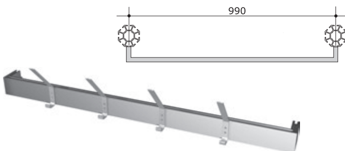
Garderobenleiste, beidseitig mit Verbinder wardrobe rail, w/ 2 connectors, 2240g
