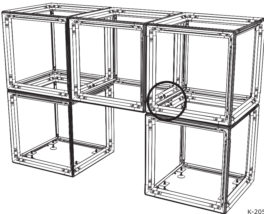
Koppelkonsole bracket to link up
