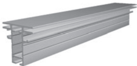
Rahmenprofil für 3mm Flach-Keder profile for frames and 3mm flat keder, 1000mm - 1367g, Herstellungslänge 6100mm production length is 6100mm
