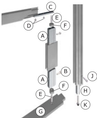
Scharnier für Universaltür hinge for universal door
