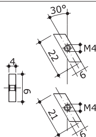
Nutenstein M4, Stahl, 3g, zum nachträglichen Einbau, für alle Nuten geeignet grooved guide M4, steel, 3g, for a later fitting in all grooves
