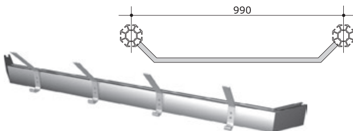
Garderobenleiste, beidseitig mit Verbinder wardrobe rail, w/ 2 connectors, 2300g
